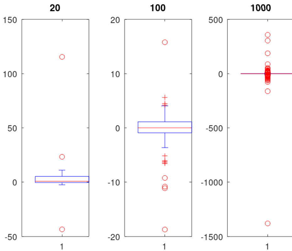
Рис. 2: Распределение Коши
